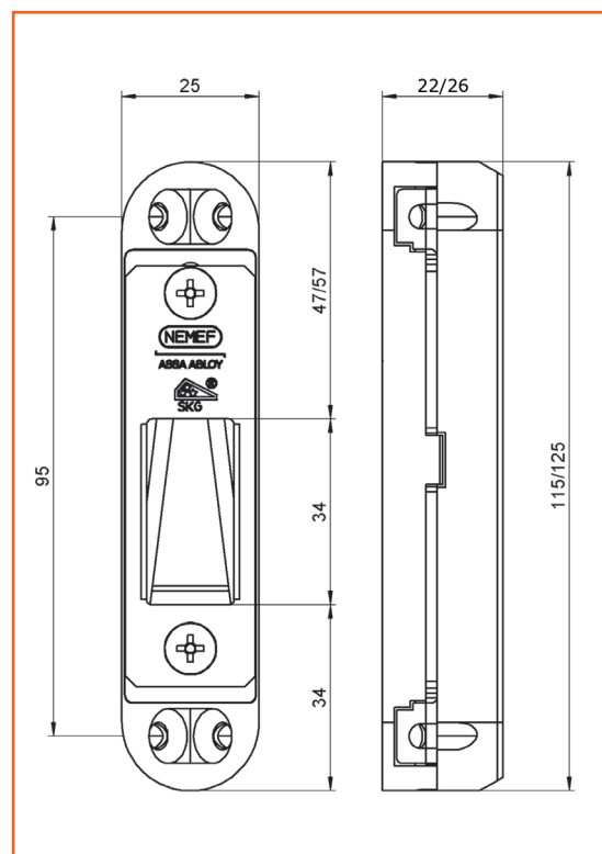
Technische tekening VS 5005 en VS 5006
